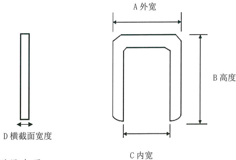
图 1: U 型卡扣外形示意图
